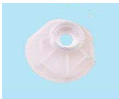
ST258003 Ø 25.8±0.1 71*71
