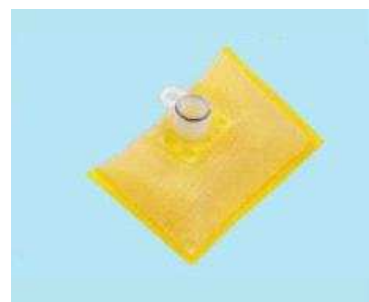
ST110056 / ST1110 Ø 11+0.1 92*62 (без пластиковой подложки)
