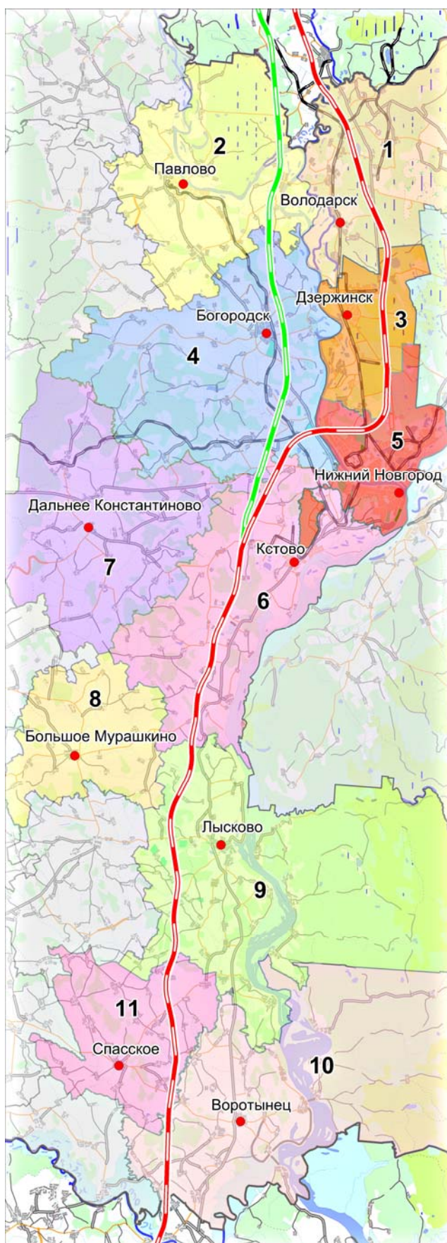
Рисунок 2.2 Схема вариантов трассы ВСМ-2 в границах Нижегородской области
