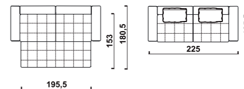
СТОУН – сборка 5
