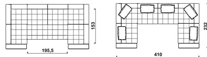
СТОУН – сборка 4
