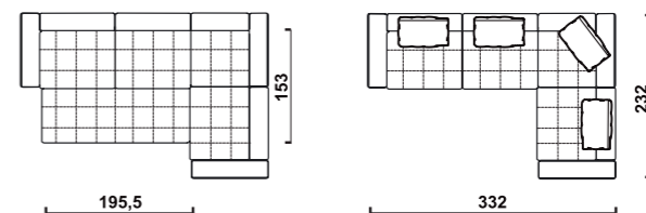
СТОУН – сборка 2
