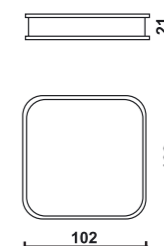
КУБА - пуф
