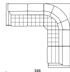
ТЕННЕССИ – сборка 8
