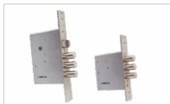
СУВАЛЬДНЫЕ ЗАМКИ ГАРДИАН Г30.11 И Г30.01
