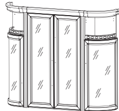
Надстройка на большой комод с балюстрадой 1780x1490x412 мм
