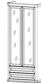
Шкаф 2-х дверный книжный 1025x2285x500 мм
