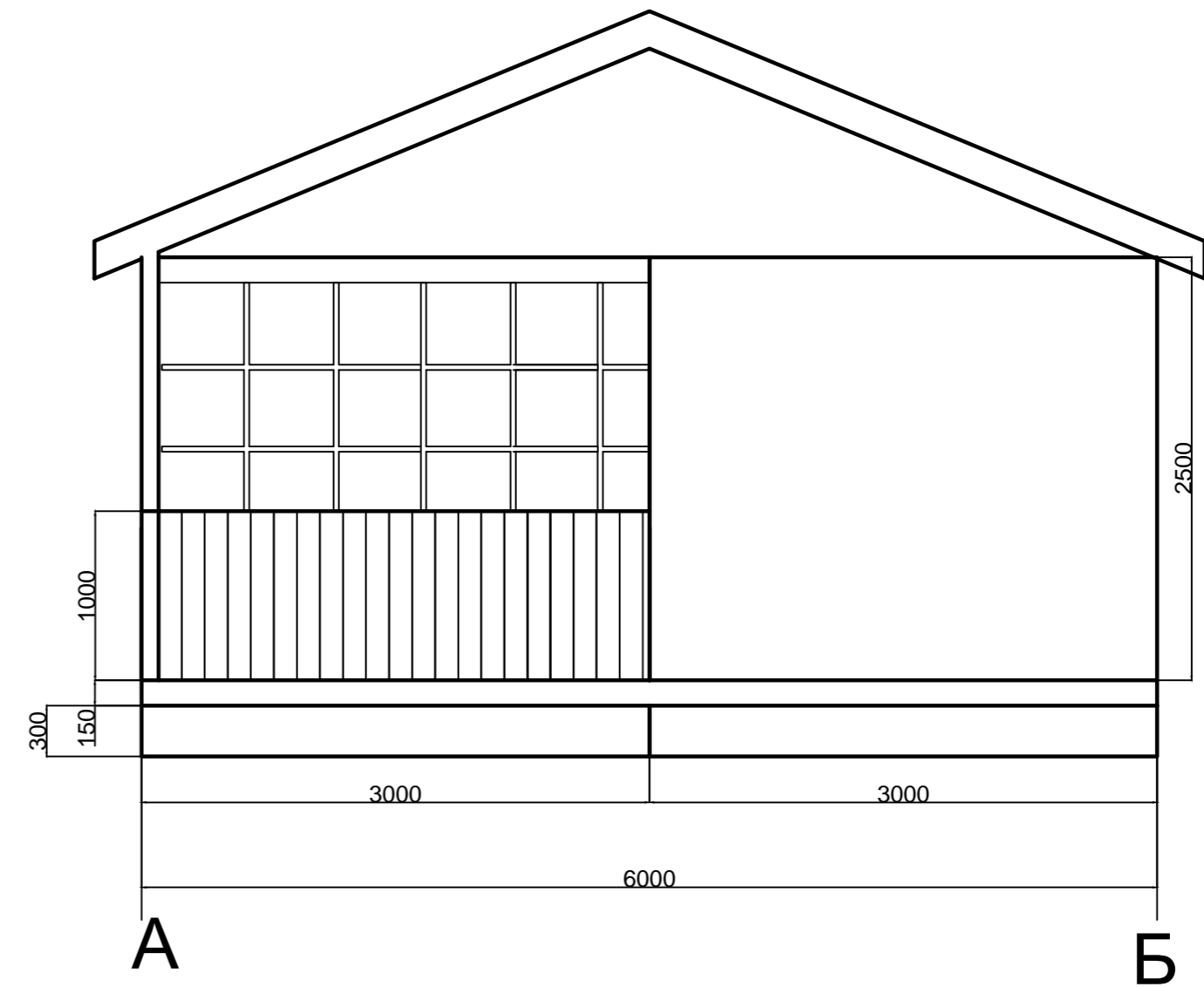
Боковой фасад в осях А-Б
