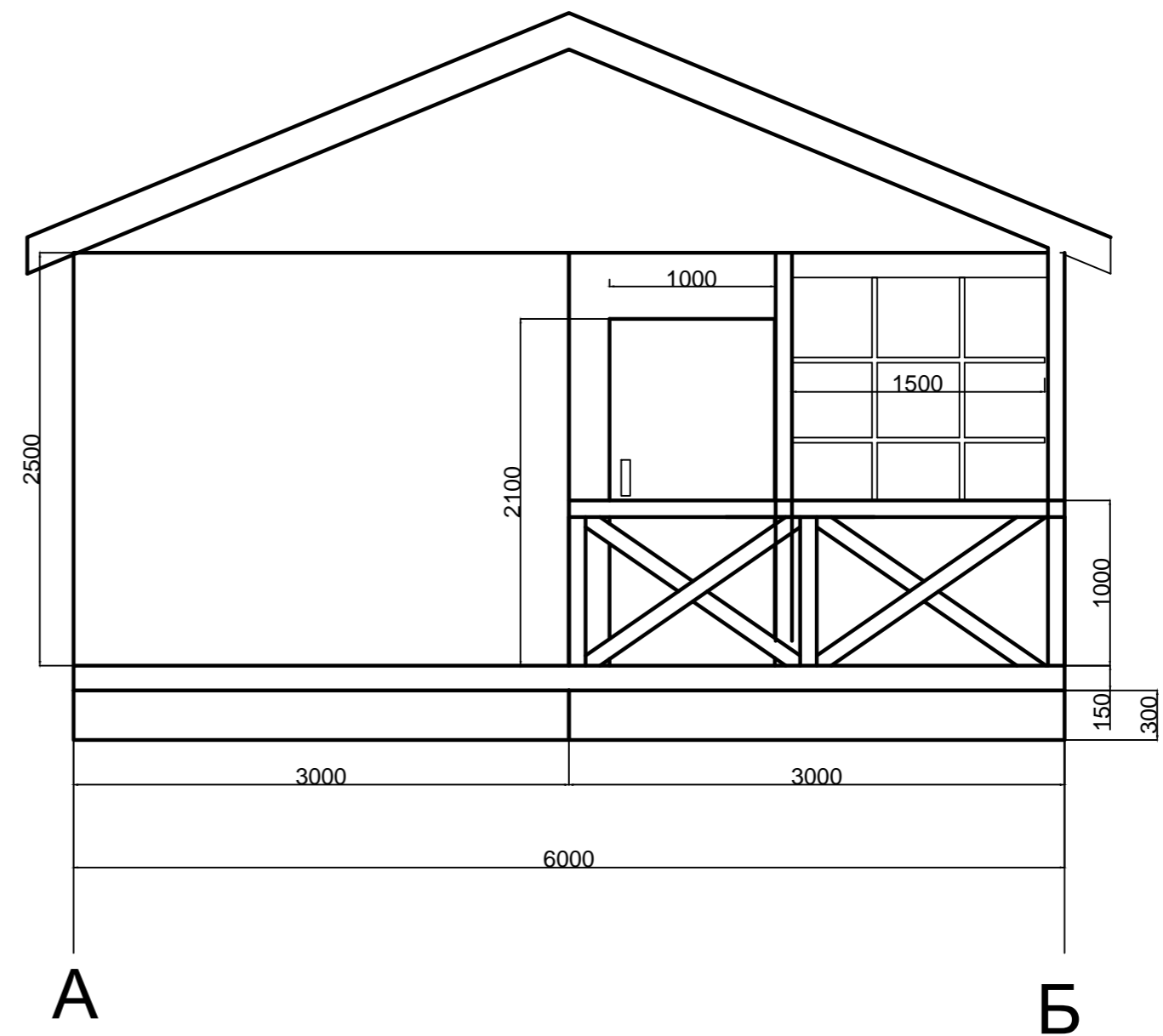
Боковой фасад в осях А-Б
