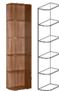
Стеллаж ШхВхГ: 320x2300x580 Собирается на левую и правую стороны 1 900.p
