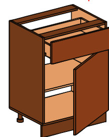
Рабочий стол РС-1Я-60 ШхВхГ: 600x846x600
