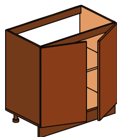
Рабочий стол РСМ-80 ШхВхГ: 800x846x600 (имеется возможность установки мойки)
