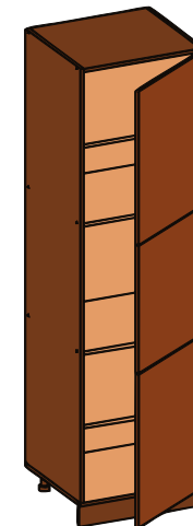
Пенал П-60 ШхВхГ: 600x2140x565 (имеется возможность установки духового шкафа)
