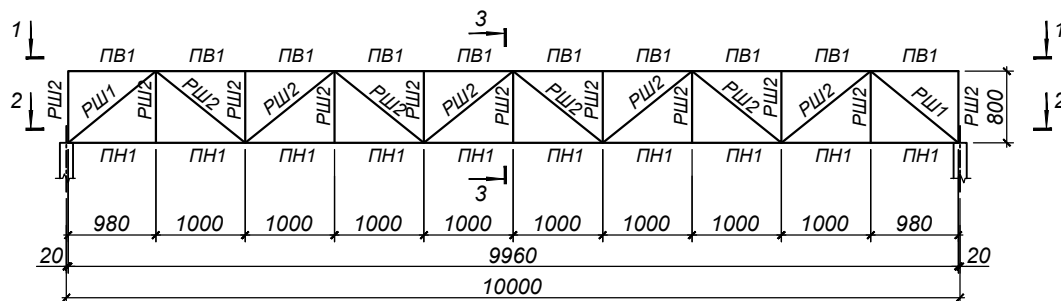
Геометрическая схема фермы ПФ2
