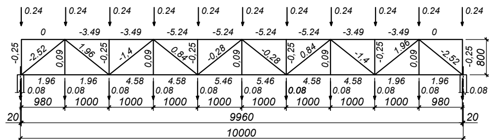
Схема усилий фермы ПФ2 (т)
