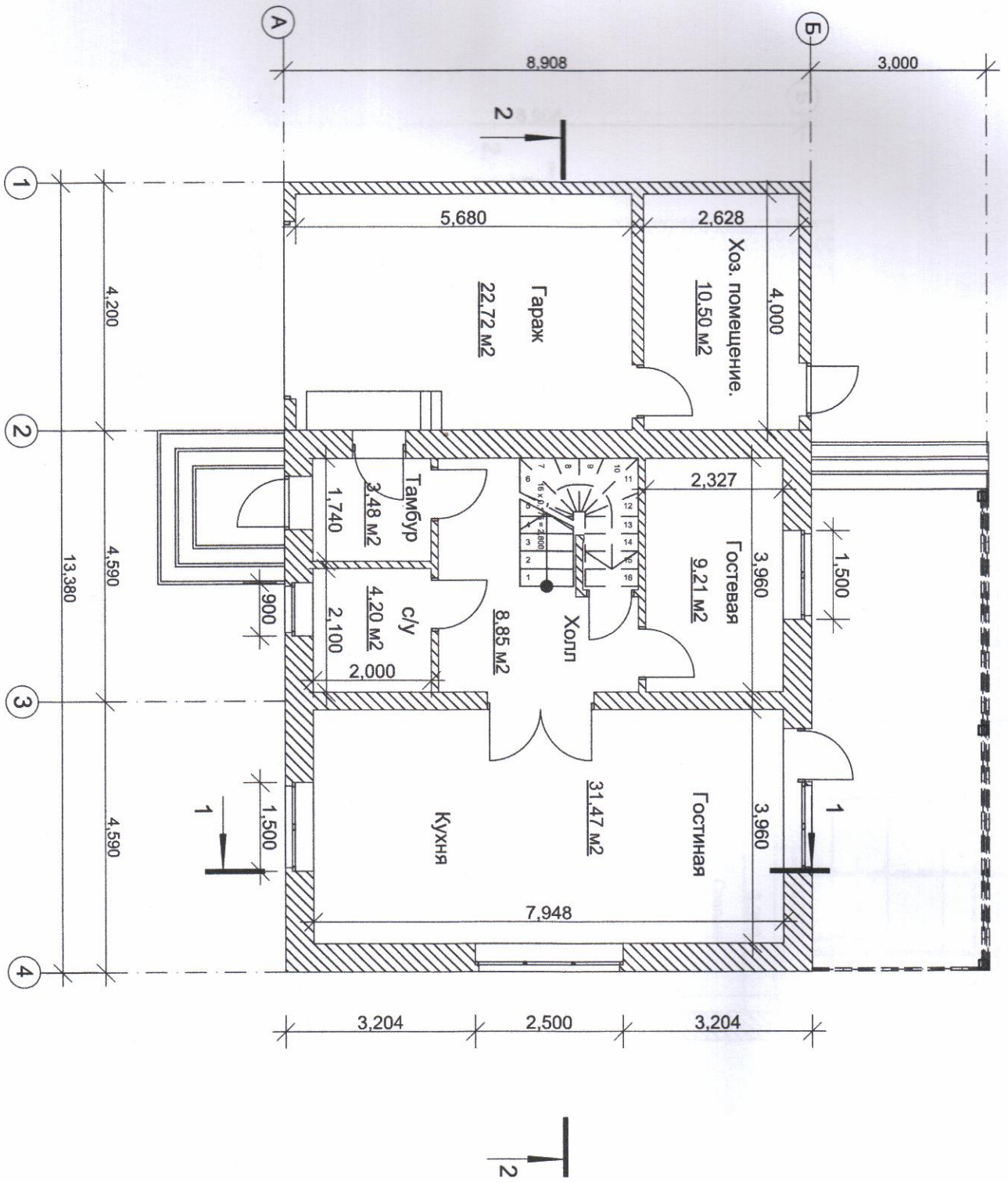
Планировка 1 этажа
