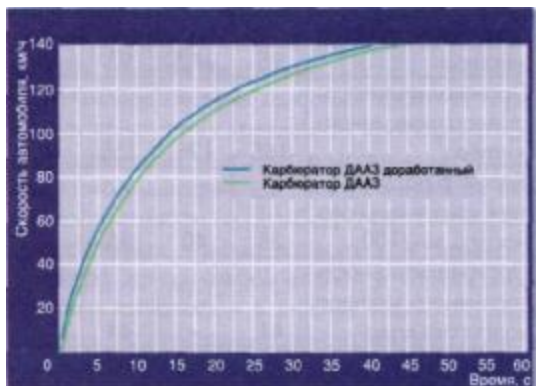
Результаты измерения разгона автомобиля ВАЗ-21093 с переключением передач до максимальной скорости
