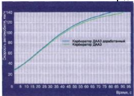
Результаты измерений разгона автомобиля ВАЗ-21093 на V передаче
