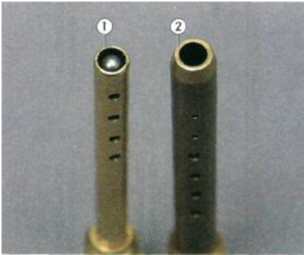
Торцы эмульсионных трубок: 1 - "ZC"; 2 - "ZD"
