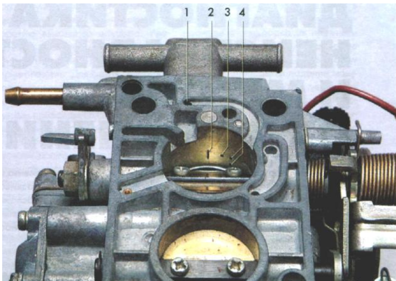
Вид на карбюратор 21073-1107010 со стороны дроссельных заслонок
