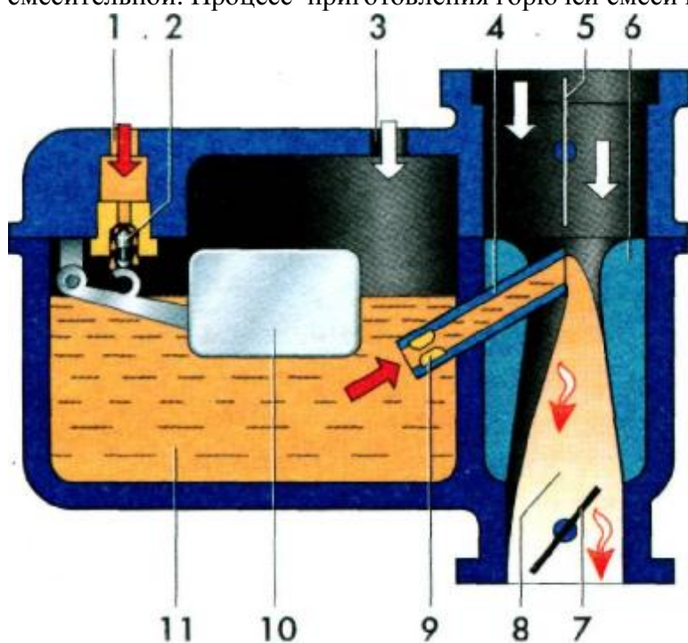
Схема простейшего карбюратора:
