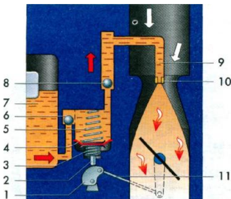
Схема диафрагменного ускорительного насоса:
