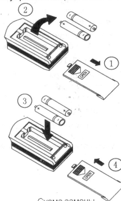
Схема замены батарей
