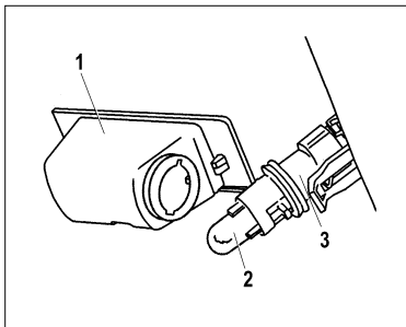
Рис. 56. Фонарь освещения номерного знака
