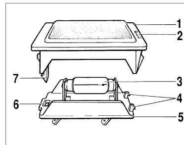
Рис. 58. Фонарь освещения вещевого ящика
