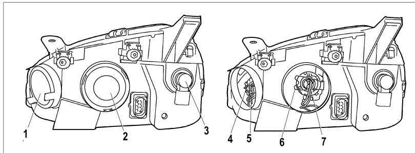
Рис. 53. Блок-фара
