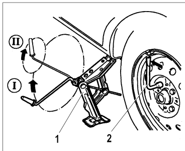
Рис. 49. Подъем автомобиля при замене колес
