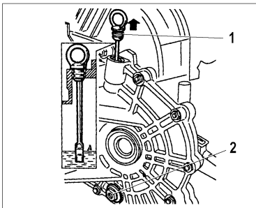
Рис. 43. Проверка уровня масла в коробке передач
