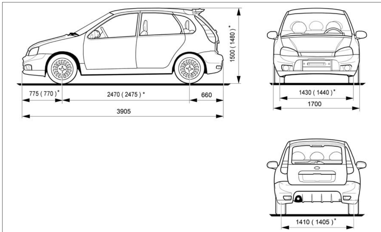
Рис. 60г. Габаритные (справочные) размеры автомобиля LADA KALINA Sport
