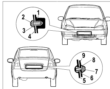
Рис. 40. Крепление номерных знаков
