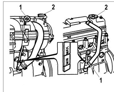
Рис. 42. Проверка уровня масла в картере двигателя
