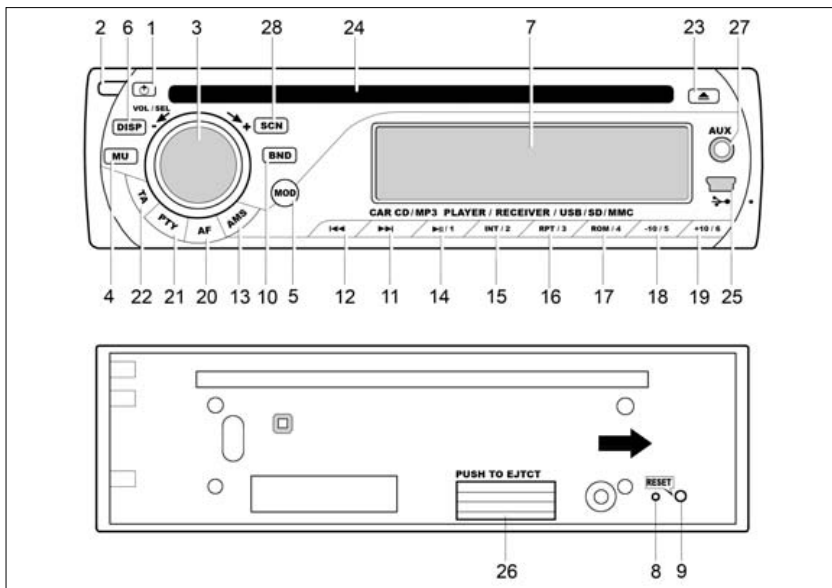
Рис. 36. Кнопки управления радиоприемником и проигрывателем компакт-дисков (при установленной и снятой передней панели)
