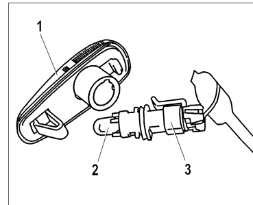
Рис. 55. Боковой указатель поворота
