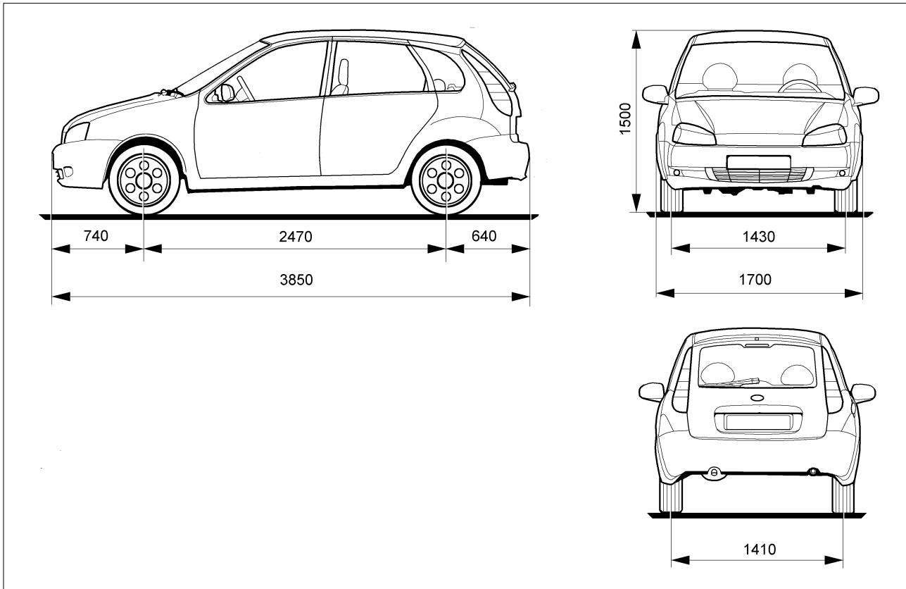
Рис. 60в. Габаритные (справочные) размеры автомобиля ВАЗ-11193 и его модификаций
