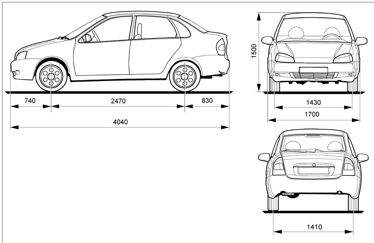
Рис. 60б. Габаритные (справочные) размеры автомобиля ВАЗ-11183 и его модификаций
