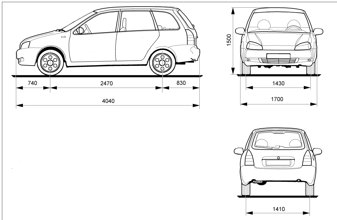
Рис. 60а. Габаритные (справочные) размеры автомобиля ВАЗ-11173 и его модификаций
